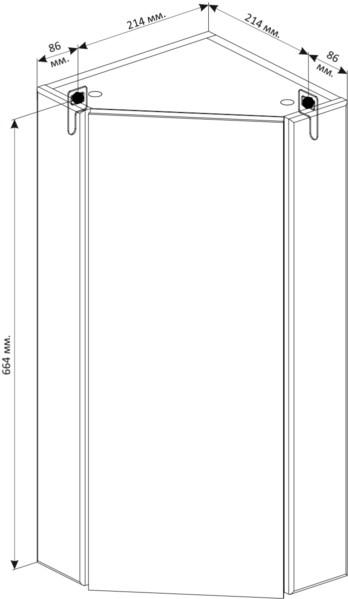
Схема навеса
